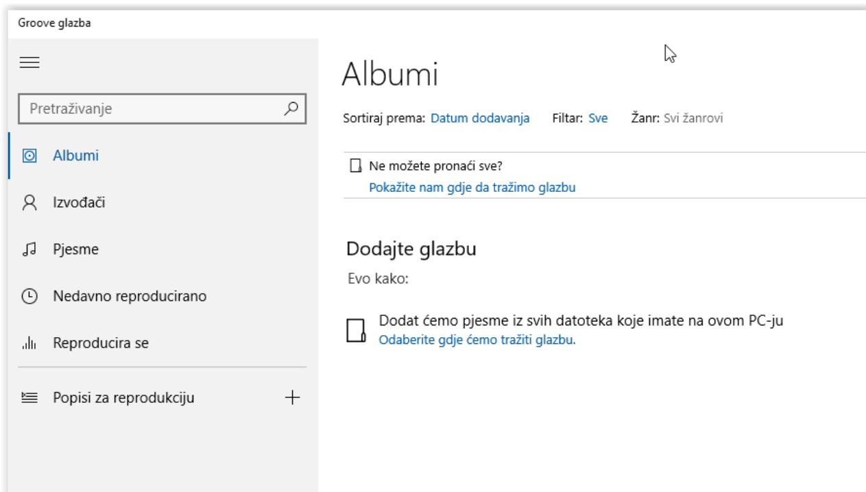
Slika 61. Aplikacija Groove
