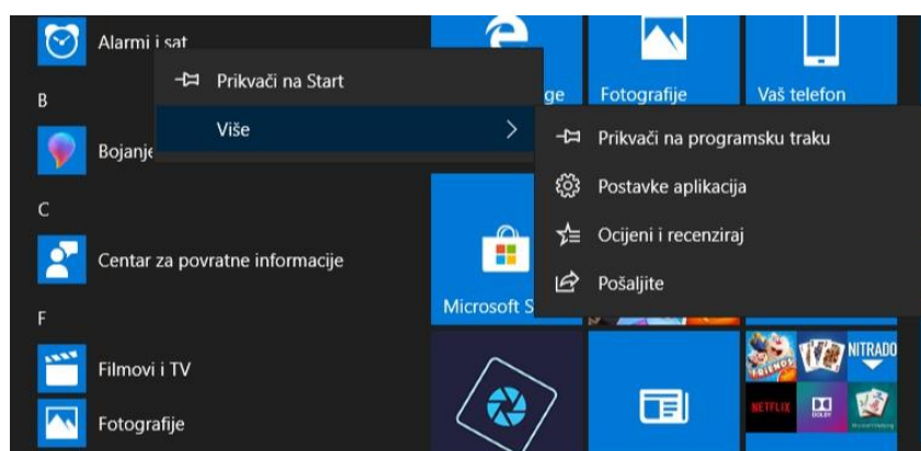
Slika 3. Mogućnosti aplikacija
