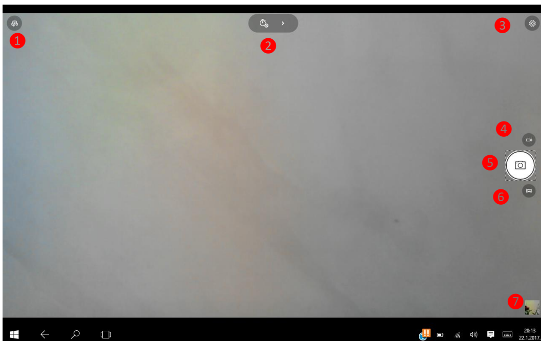
Slika 52. Aplikacija Kamera
