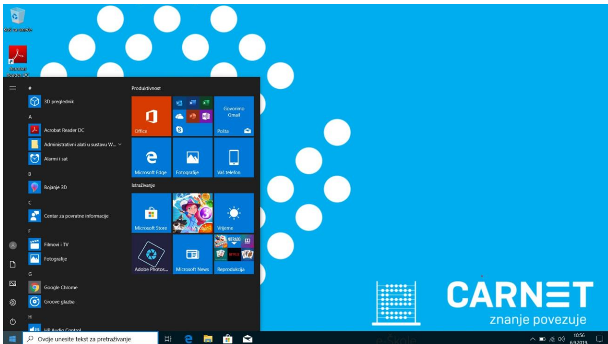
Slika 3. Početno sučelje
