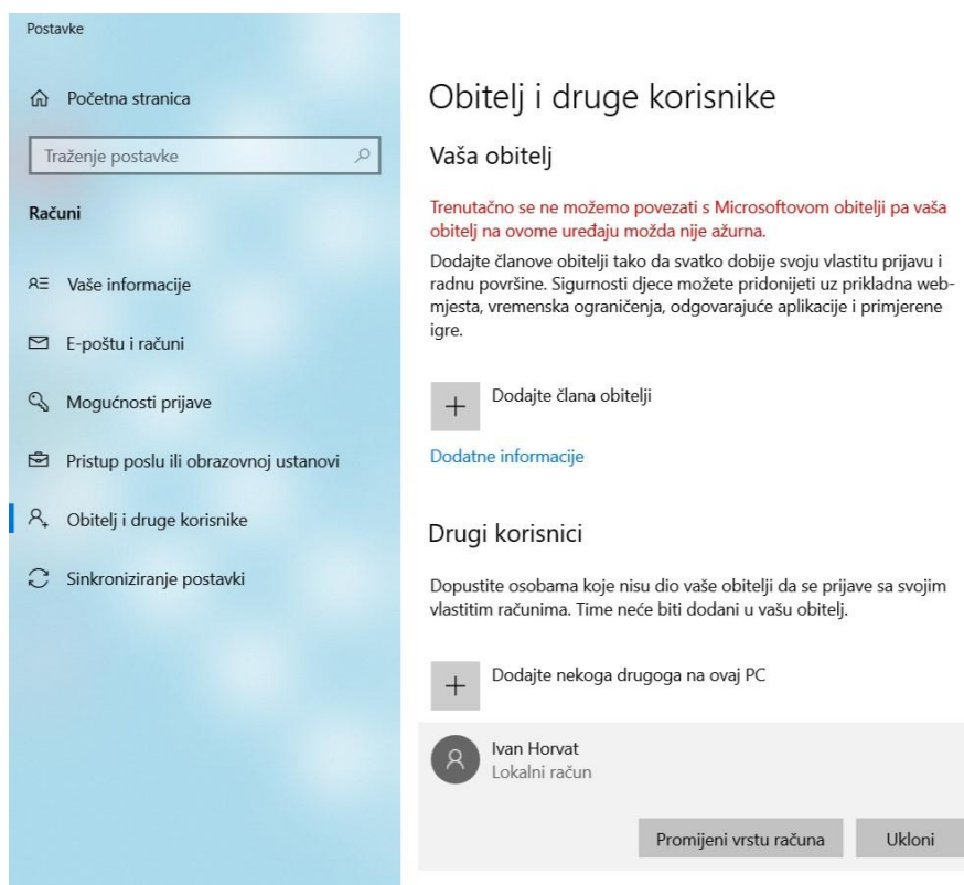
Slika 35. Odabir korisnika
