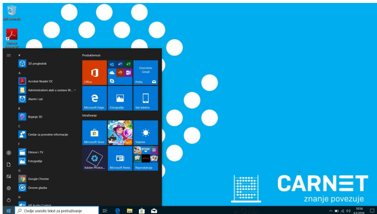
Slika 1. Izbornik Start
